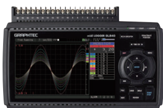
多种信号输入型 midi LOGGER GL840-M
